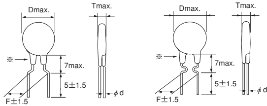
图1 (Y弯曲)
